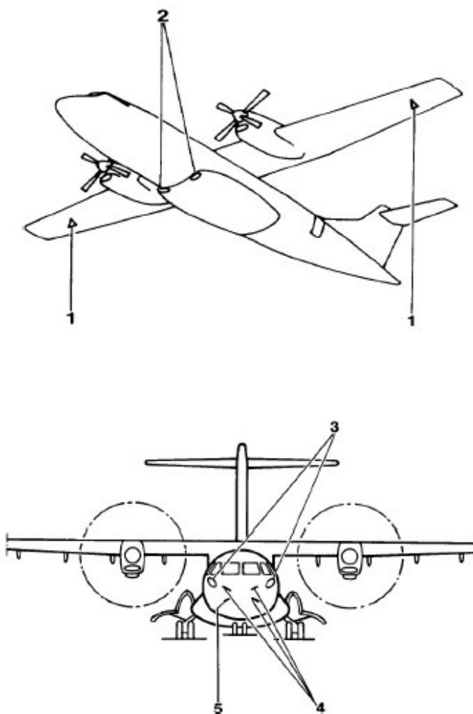
Рис. 2 – Установка заглушек и защитного оборудования на АTR-42/72
